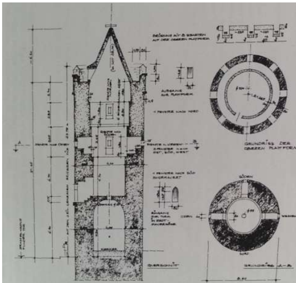
Bild [11]: Skizze eines Schnittes und Grundriss
